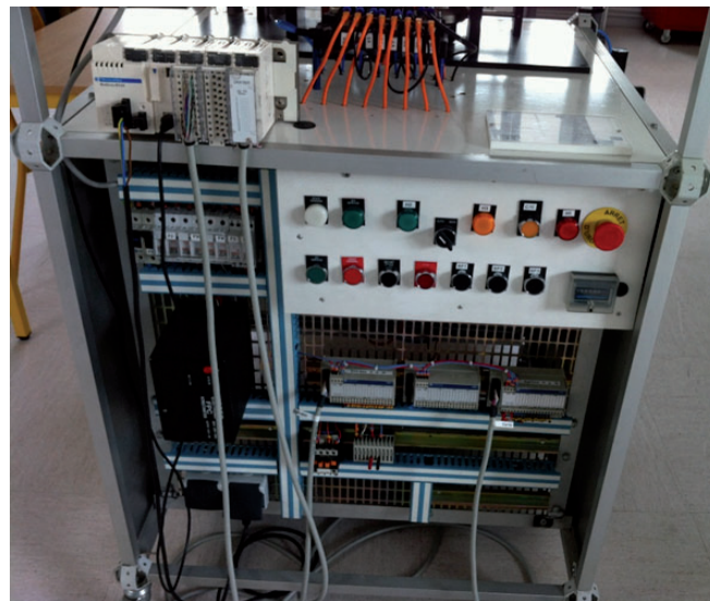
Armoire avec automate Schneider et ces connecteurs de raccordement.
