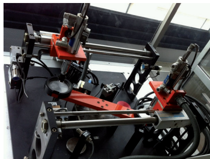
La partie opérative permet la préhension des pièces et le transfert sur différents postes à l'aide d'un vérin rotatif.
