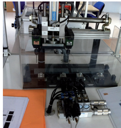
Cette machine permet le perçage de 2 pièces simultanément, l'unité de perçage est montée sur un système mobile qui permet après déplacement de percer 2 autres pièces.
