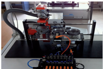
La partie opérative permet la préhension des pièces et le transfert sur différents postes.
