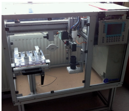
L'ensemble de la machine est géré par un automate SIEMENS ET200S CPU + coupleur Profibus Dp. Le déplacement de l'axe horizontal pour aller se positionner au-dessus des ampoules avant la préhension est piloté par un moteur brushless commandé depuis le réseau Profibus DP. Le pupitre permet des formations sur le logiciel Winccflexible.
